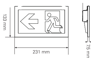
Montagem saliente de tecto
