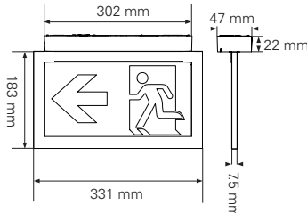
Montagem saliente de tecto
